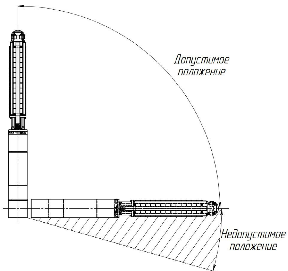
Рис. 8 Условия для горизонтального монтажа
