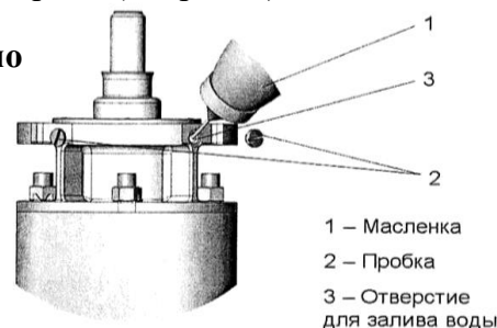
Рис. 3 Схема доливки воды
