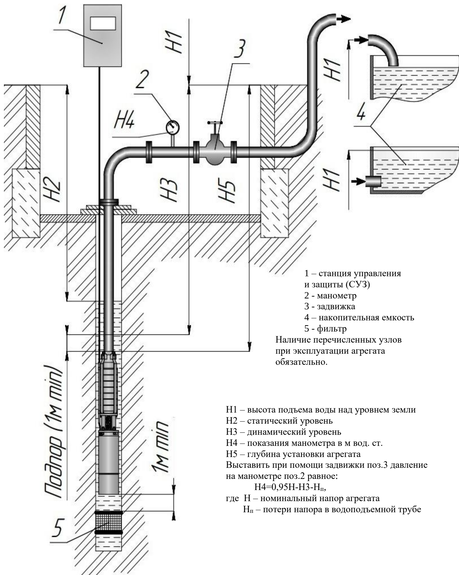
Рис. 6 Схема монтажа агрегата с указанием высот для заполнения листа «Сведения об условиях эксплуатации»
